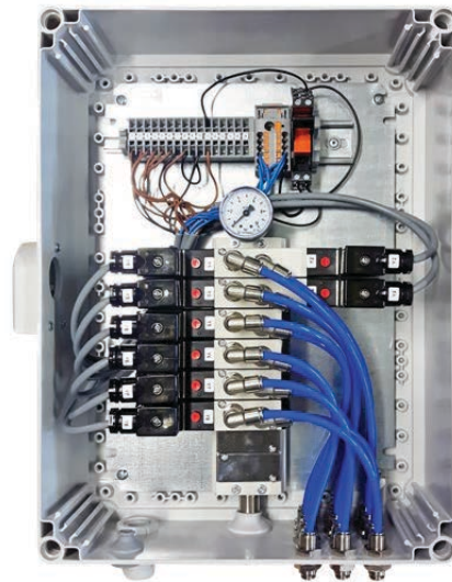
Venttiilikokoonpanot
